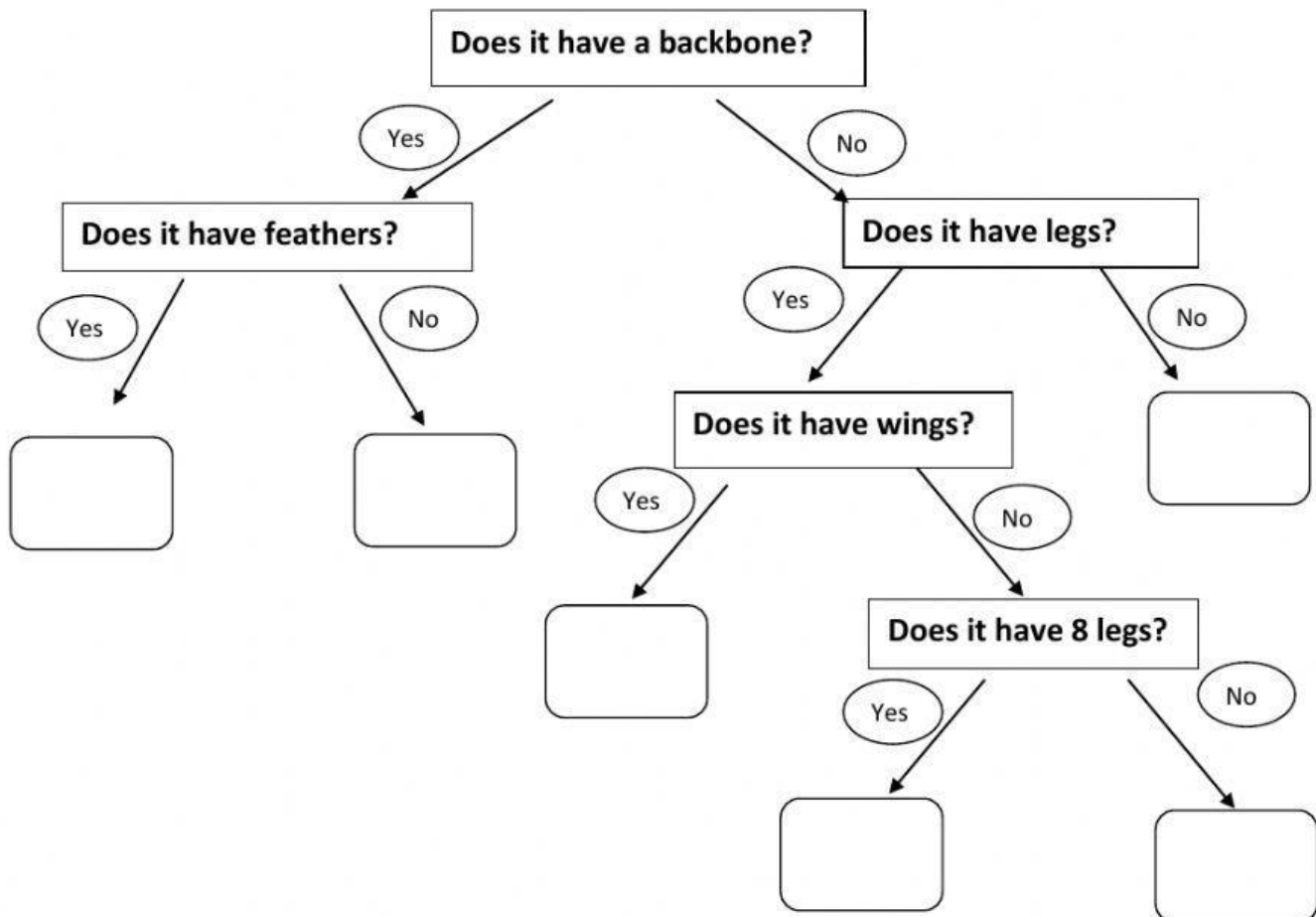
worm
