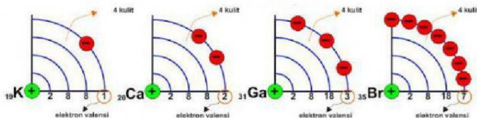
Gambar 3. Ilustrasi Jari-jari Atom dalam Satu Periode.
