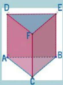
Prisma segitiga
