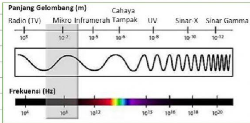
Gambar 6. Rentang Spektrum Gelombang Elektromagnetik
