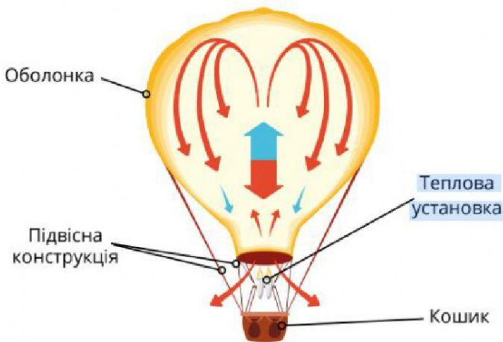
Будова аеростата
