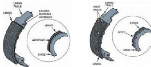
Gambar 1. 9 Sepatu rem
