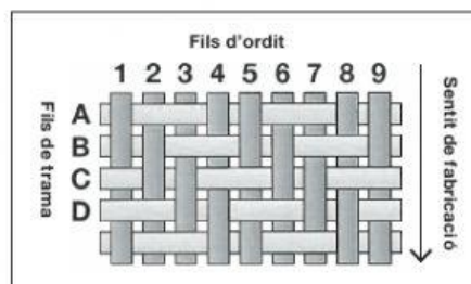
Estructura d'una sarja
