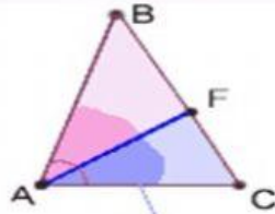
[A F] – биссектриса треугольника ABC
