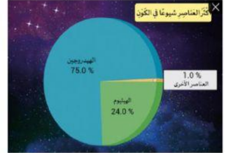
الشكل (أ) العناصر أكثر شيوعاً في الكون
