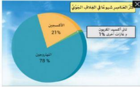
الشكل ( ب ) العناصر أكثر شيوعاً في الغلاف الجوي
