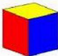
Cubo (Hexaedro)
