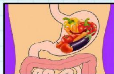
Digestión
