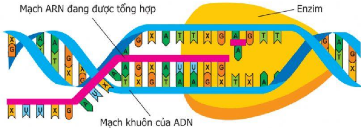
Hình 17.2. Sơ đồ tổng hợp phân tử ARN
