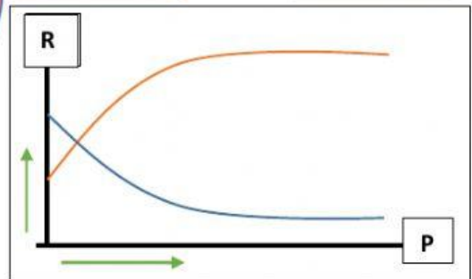
Gambar : Grafik Laju Reaksi perubahan konsentrasi produk dan konsentrasi reaktan
