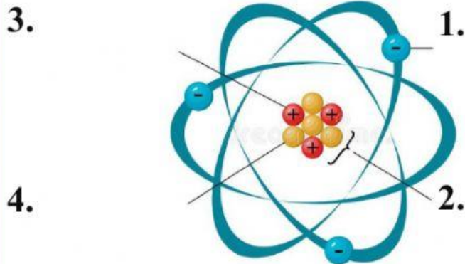
Cấu tạo nguyên tử
