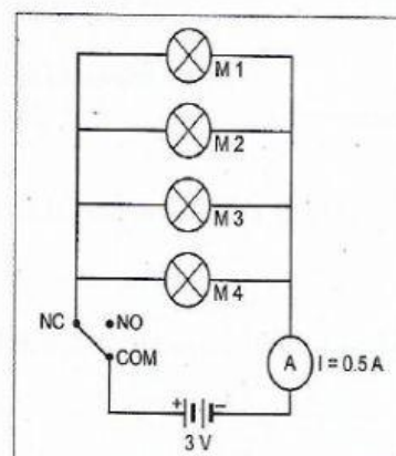
Litar B
