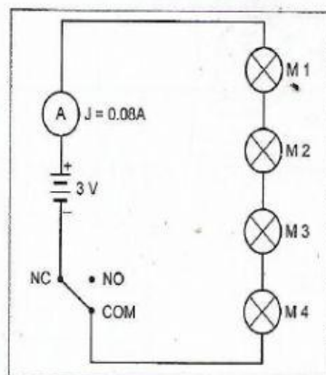
Litar A
