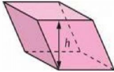
Prisma oblicuo
