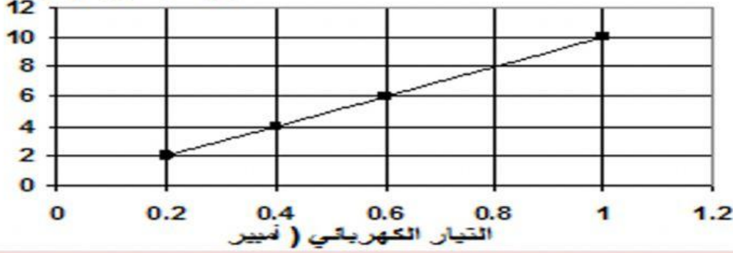
جهد البطارية ( فولت )
