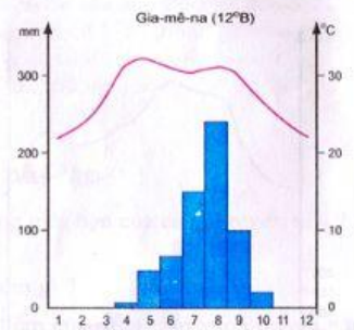
Hình 6.2 - Biểu đồ nhiệt độ và lượng mưa ở Gia-mê-na (Sát)
