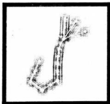
Buruj Skorpio
