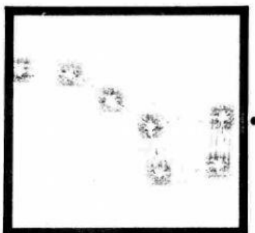
Buruj Biduk
