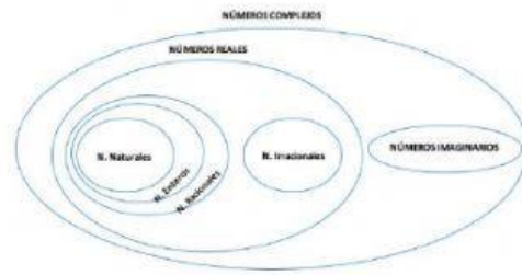
Esquema de los números complejos
