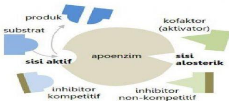
Gambar 1. Struktur Enzim Sumber : materibelajar.co.id
