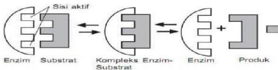
Gambar. 2 Teori Lock and Key Sumber: Dunia Pendidikan
