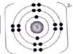
Ion sulfida (2.8.8) Sulphide ion (2.8.8)
