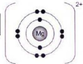
Ion magnesium (2.8) Magnesium ion (2.8)
