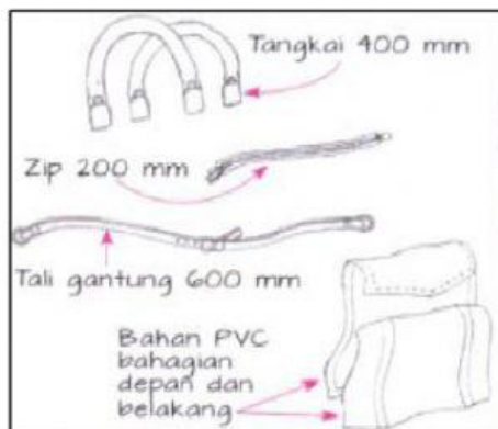
Rajah 2 : Lakaran ceraian
