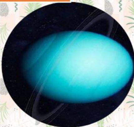
8. Uranus
