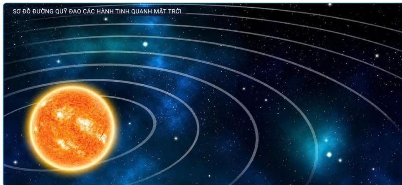
HÌNH ẢNH 8 HÀNH TINH TRONG HỆ MẶT TRỜI (THEO THỨ TỰ)
