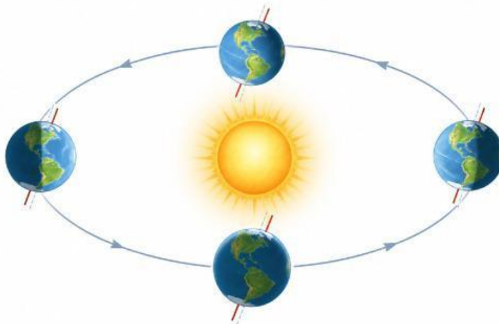
Schéma obehu Zeme okolo Slnka a striedania ročných období
