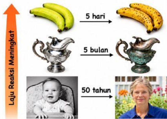
Gambar 4. Contoh reaksi kimia dalam kehidupan Sumber: Kusuma (2023, hlm. 157)
