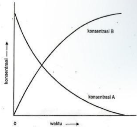
Gambar 3. Grafik perubahan konsentrasi reaktan menjadi produk setiap satuan waktu. Sumber: Syukri (1999, hlm. 469).
