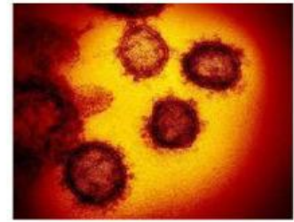
Gambar 1. 1 Mikroskopis Virus corona
