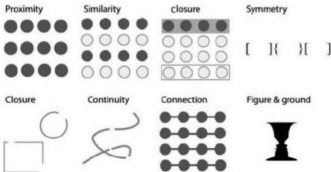
Рис. 7. Принципи гештальту
