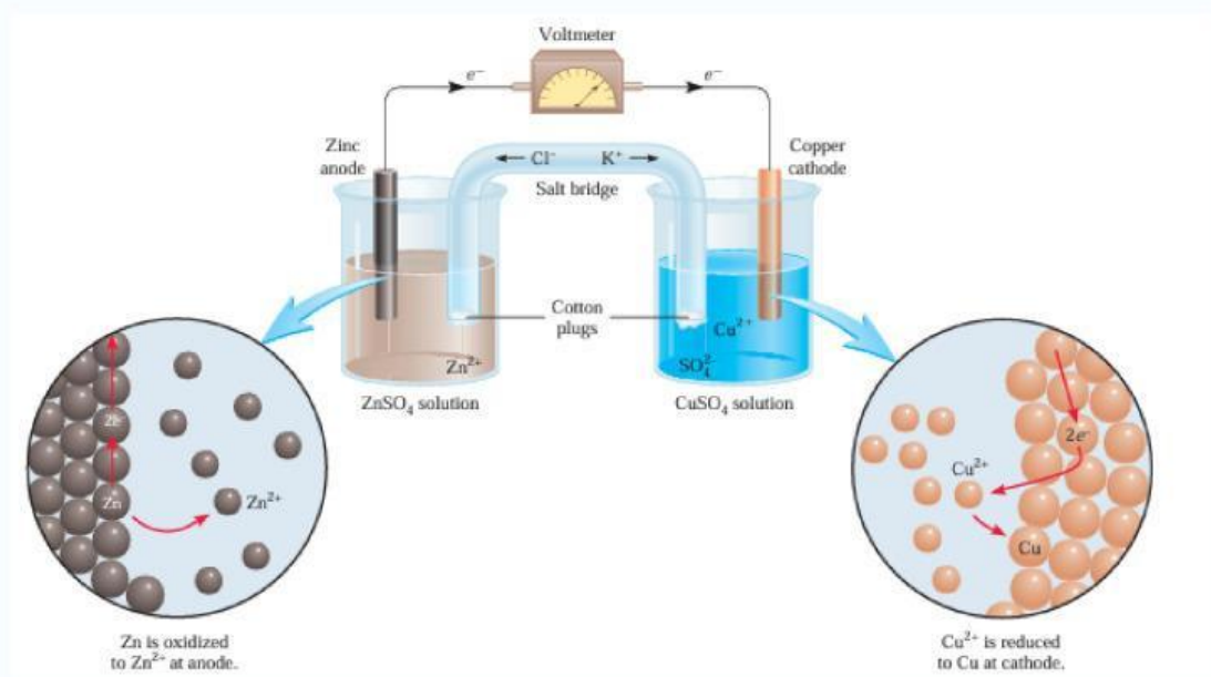
Gambar. Diagram Sel Volta
