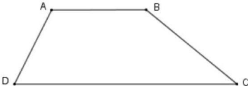
Hình thang ABCD
