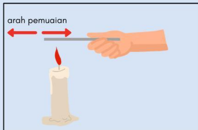
Gambar 1. Batang logam memuai saat dipanaskan
