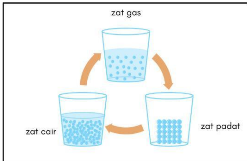
Gambar 2. Susunan partikel zat padat, cair, dan gas
