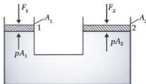
Gambar. prinsip kerja dongkrak hidrolik dalam hukum pascal
