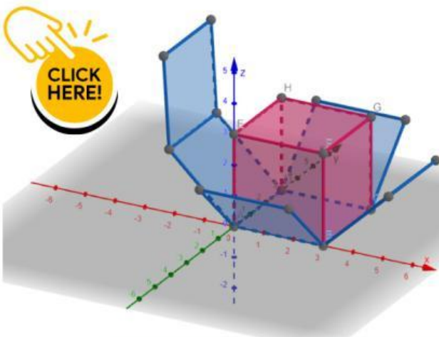
Gambar 1.9. Jaring-jaring kubus di GeoGebra
