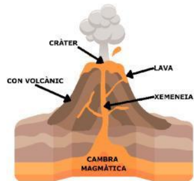
Figura 1. Parts d'un volcà
