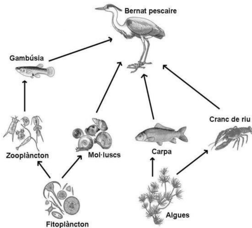
Figura 4. Xarxa tròfica d'un riu europeu
