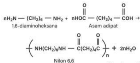
Gambar 2. 2 Pembentukan nylon-66
