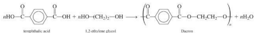
Gambar 1. 11 Pembentukan Poliester
