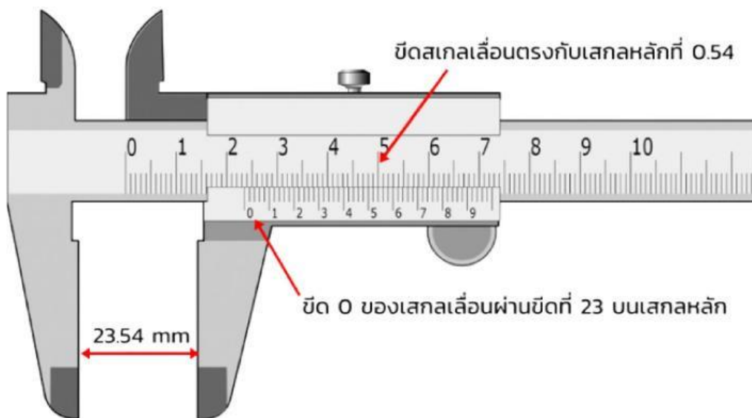
รูปที่ 8 การอ่านค่าเวอร์เนียคาลิปเปอร์ ค่าความละเอียด 1/50 มิลลิเมตร (0.02 มิลลิเมตร)
