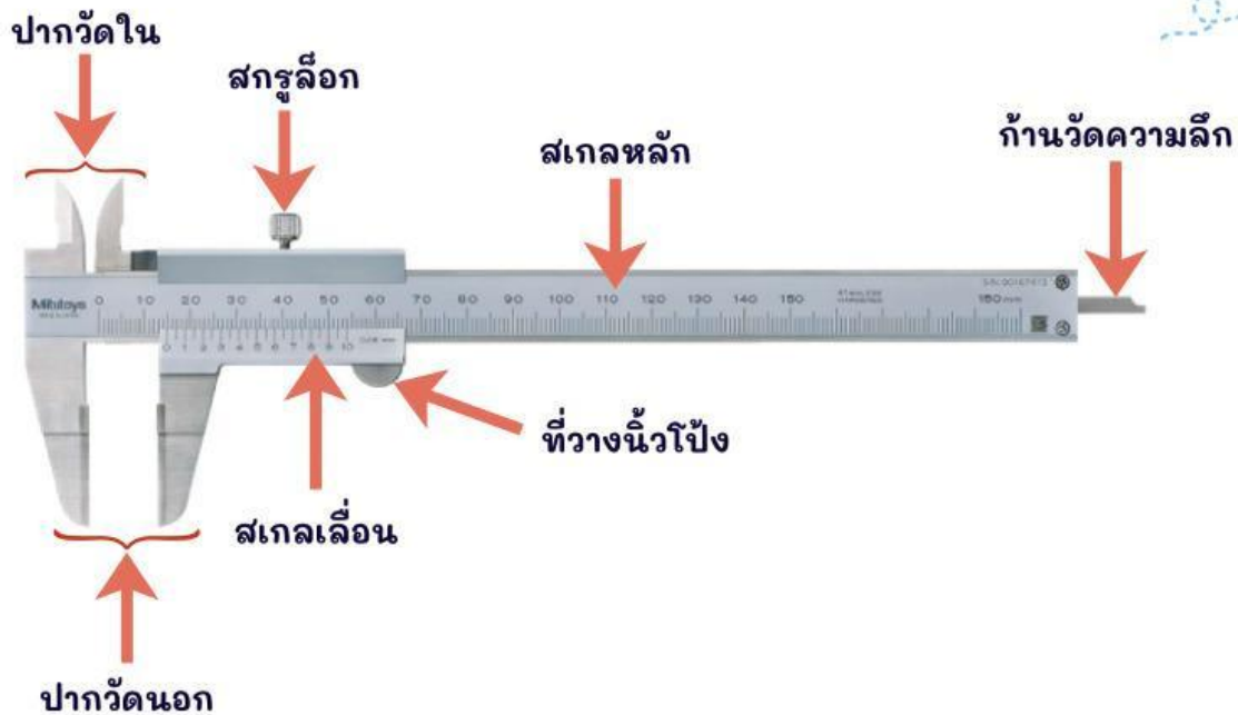
รูปที่ 4 ส่วนประกอบของเวอร์เนียคาลิเปอร์แบบอนาล็อก
