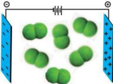
مولکولهای F 2
