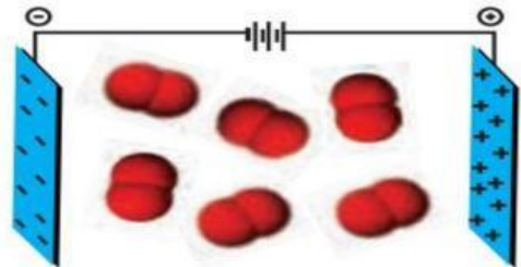
مولکول های O 2
