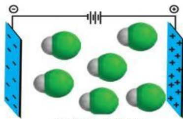
جهت گیری مولکول های HCl در میدان الکتریکی
