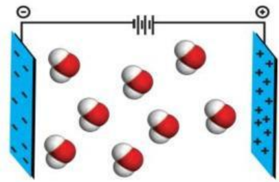
شکل ۱۵- جهت گیری مولکول های آب در میدان الکتریکی
