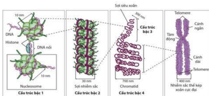
Sơ đồ các bậc cấu trúc siêu hiển vi của nhiễm sắc thể
