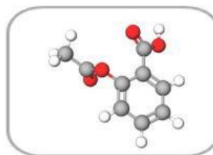
Slika 3: Slika krogljčnega modela molekule acetilsalicilne kisline (povezava do interakt. prikaza)
