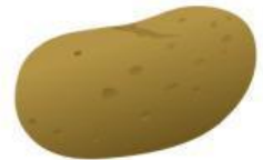
potato
