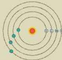
Atom Bohr
