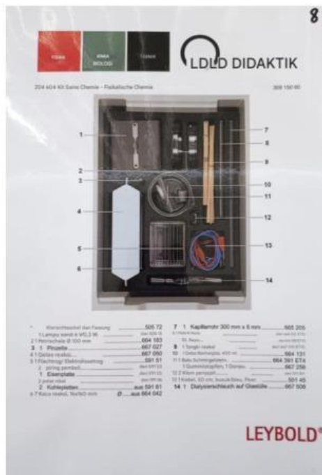
Gambar 2. Daftar Alat KIT Laboratorium Sel Elektrolisis
