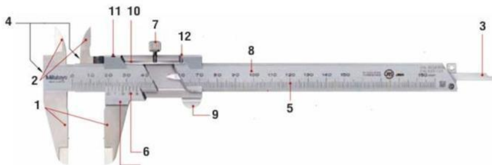
รูปที่ 3-5 ส่วนประกอบของเวอร์เนียคาลิเปอร์
