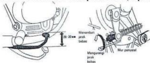
Gambar 5. 15 Penyetel Jarak Main Bebas Pedal
