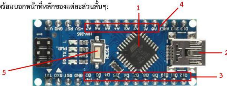
(ภาพที่ 1: รูปร่างบอร์ด Arduino Nano ที่มีหมายเลขชี้ไปยังส่วนประกอบต่างๆ)
