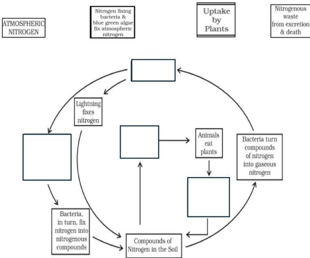
Fig. 2.10 : Nitrogen cycle
