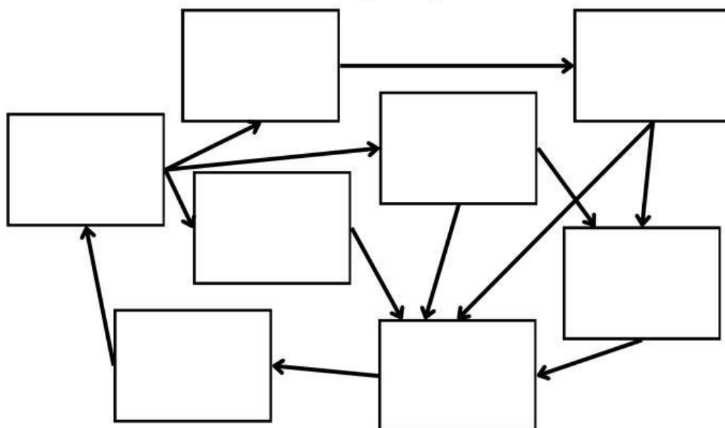
Skema Jaring-Jaring Makanan
