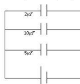
rangkaian paralel
