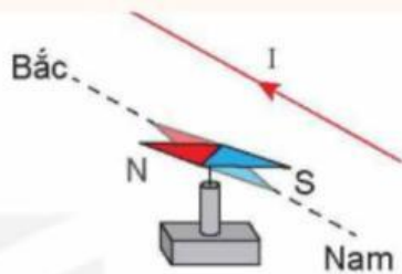
Hình 14.2. Thí nghiệm của Oersted (Ơ-xtét) về tương tác giữa dòng điện và kim nam châm
