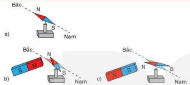
Hình 14.1. Thí nghiệm về tương tác giữa nam châm với kim nam châm a) Kim nam châm tự do b) Khi hai cực cùng tên lại gần nhau c) Khi hai cực khác tên lại gần nhau
